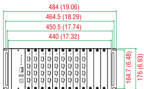
主视图
