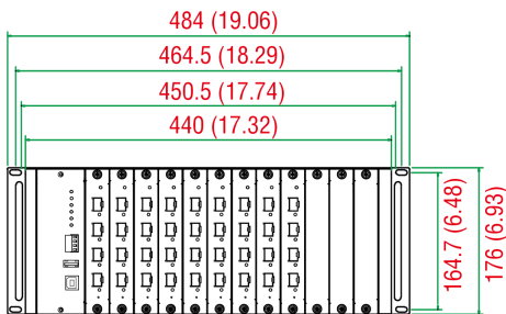
主视图
