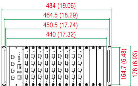
前视图
