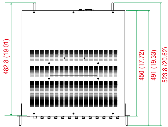
俯视图
