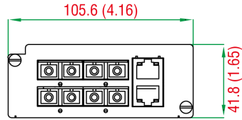
主视图
