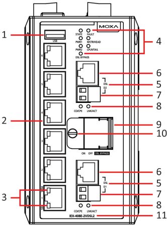
IEX-408E-2VDSL2-HV
