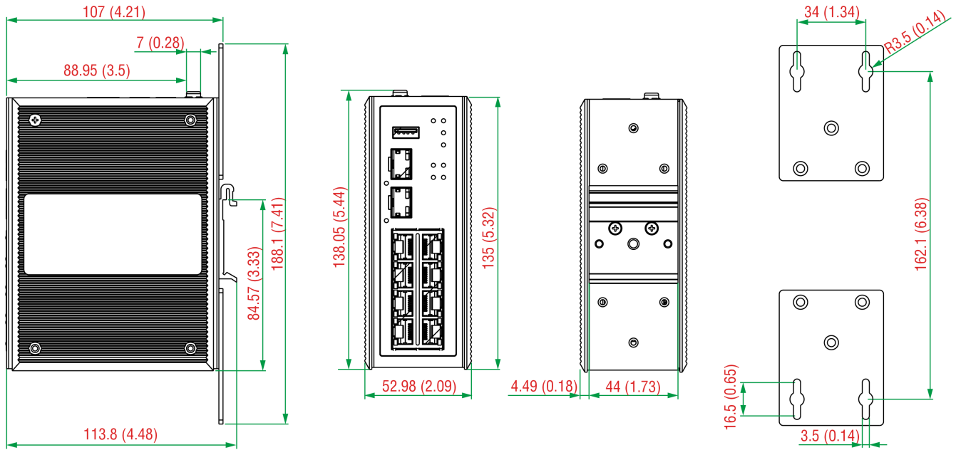
侧视图
